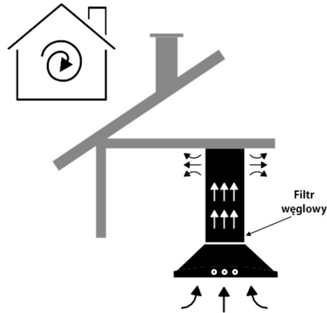
Obr. 4. Digestoř jako odsavač kanystřů
