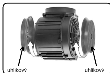
Obr. 9. Montáž a demontáž uhlíkových filtrů na turbíně
