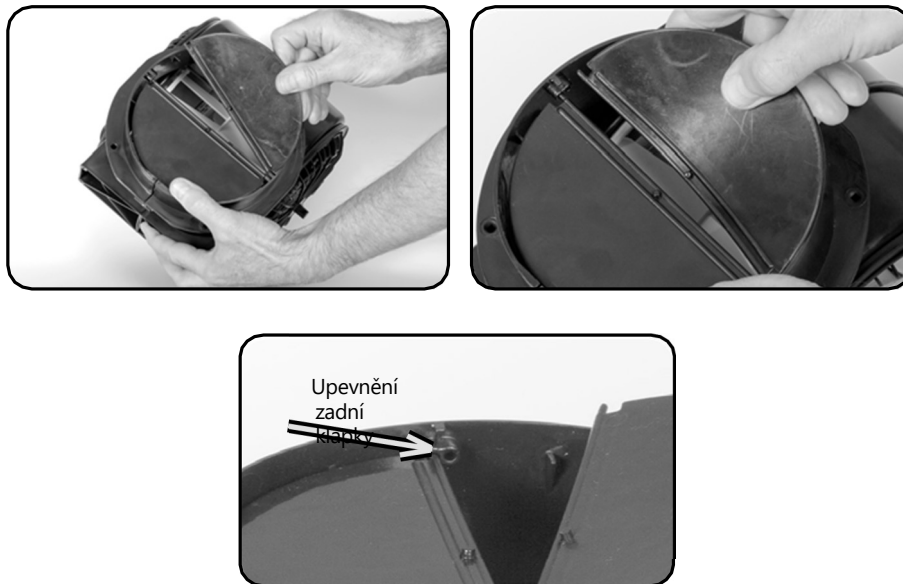
Obr. 4. Instalace zpětných klapek na výstupu z turbíny
